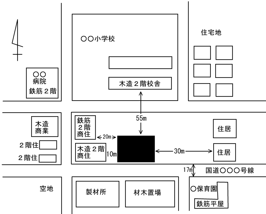
機械施設の配置図
